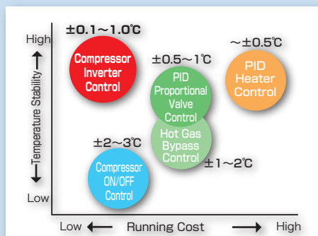
(RKE1500B1-V, B1-VW)
